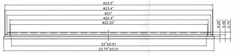
魚雷發射管外門迫緊圖 S:6=1'-0"
